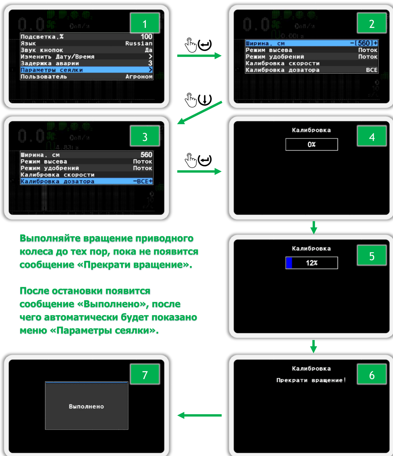
Рисунок 37 Калибровка дозатора
